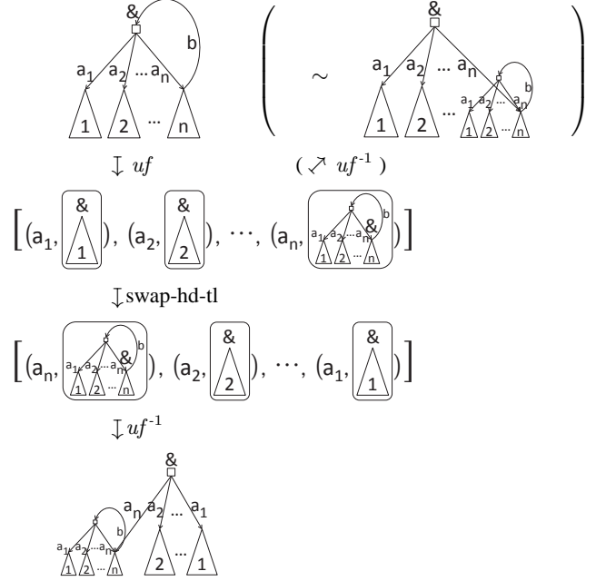
Figure 8. \mathbf{l-sbl}(\text{swap-hd-tl}) (= uf^{-1} \circ \text{swap-hd-tl} \circ uf)
